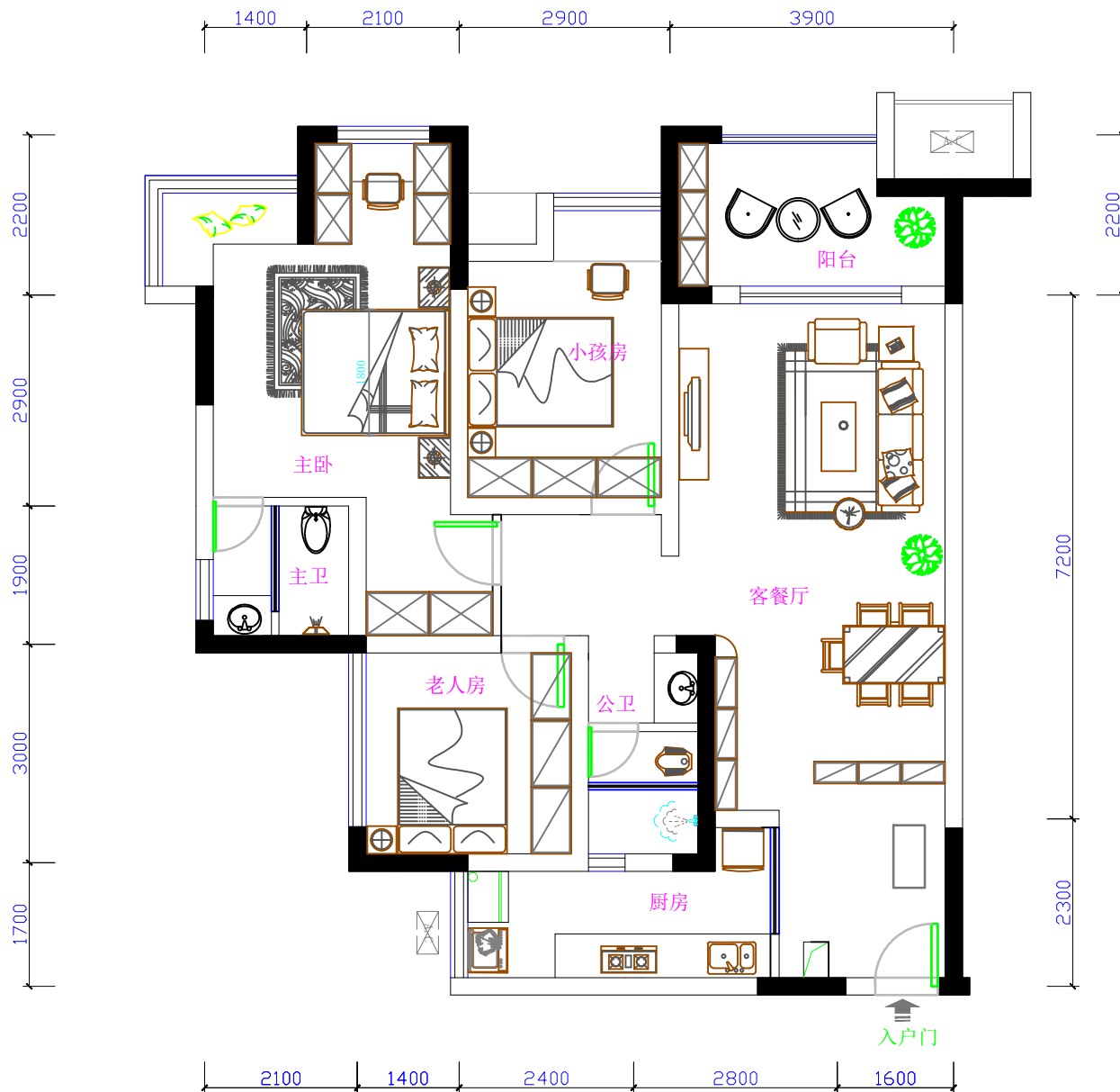
平面布局图 1: 100
