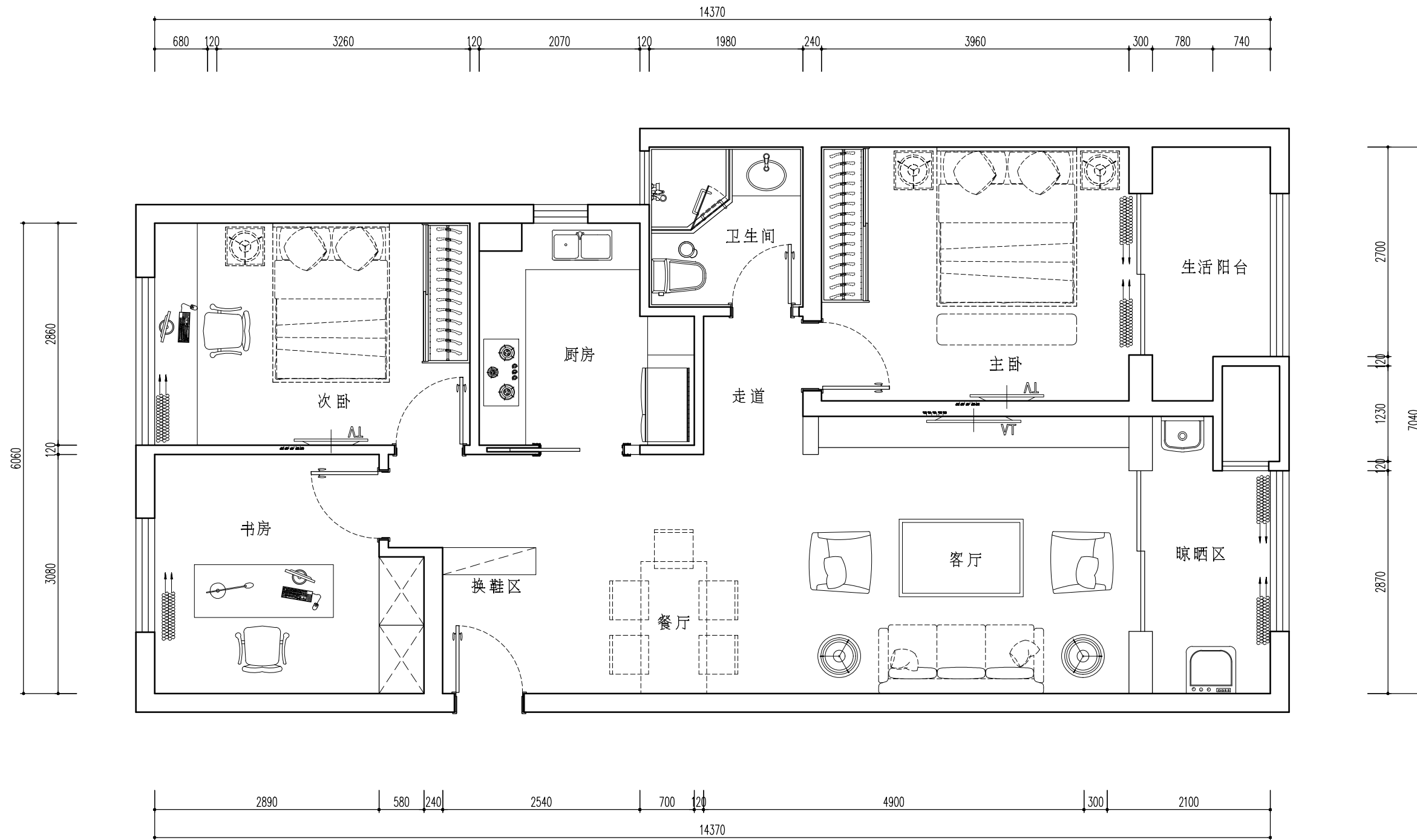
2F PLAN 平面布置图 SCALE: 1:40
