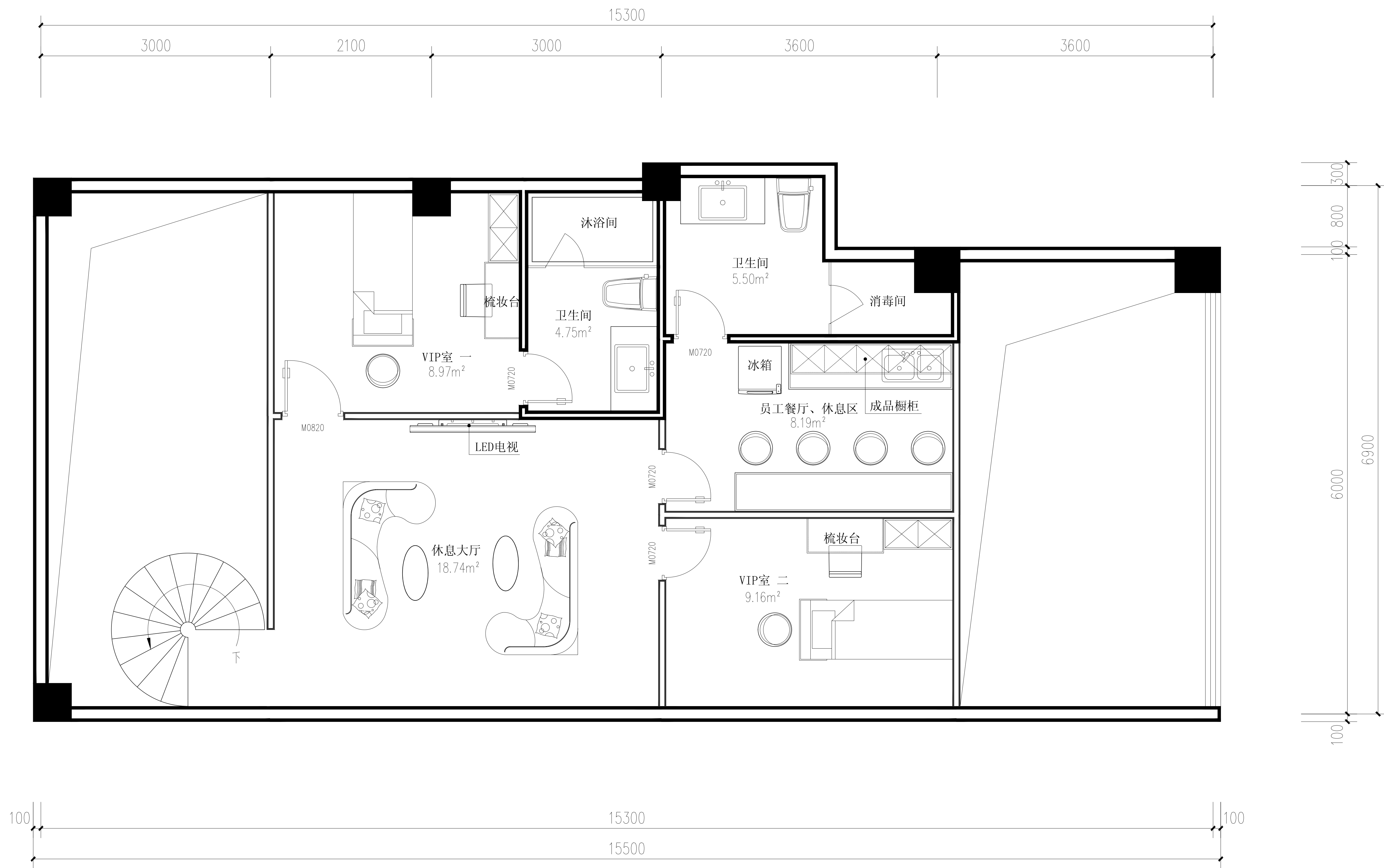
夹层平面布置图 1:50
