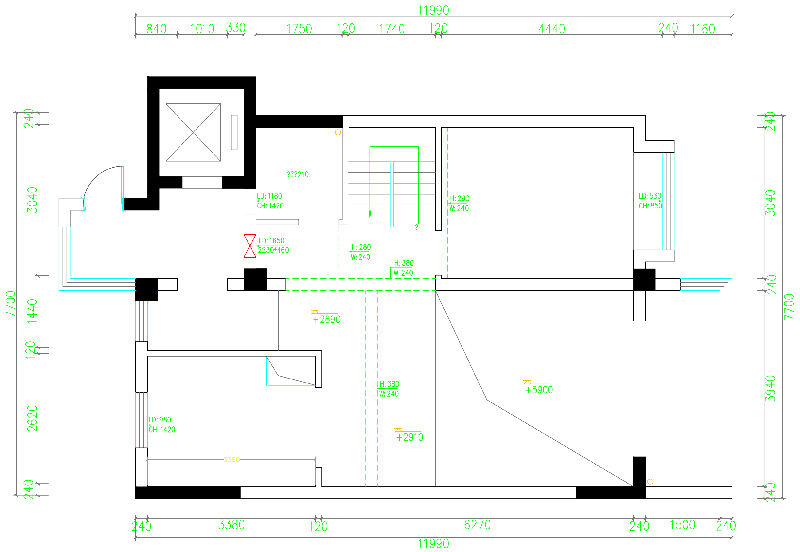
原始结构图
